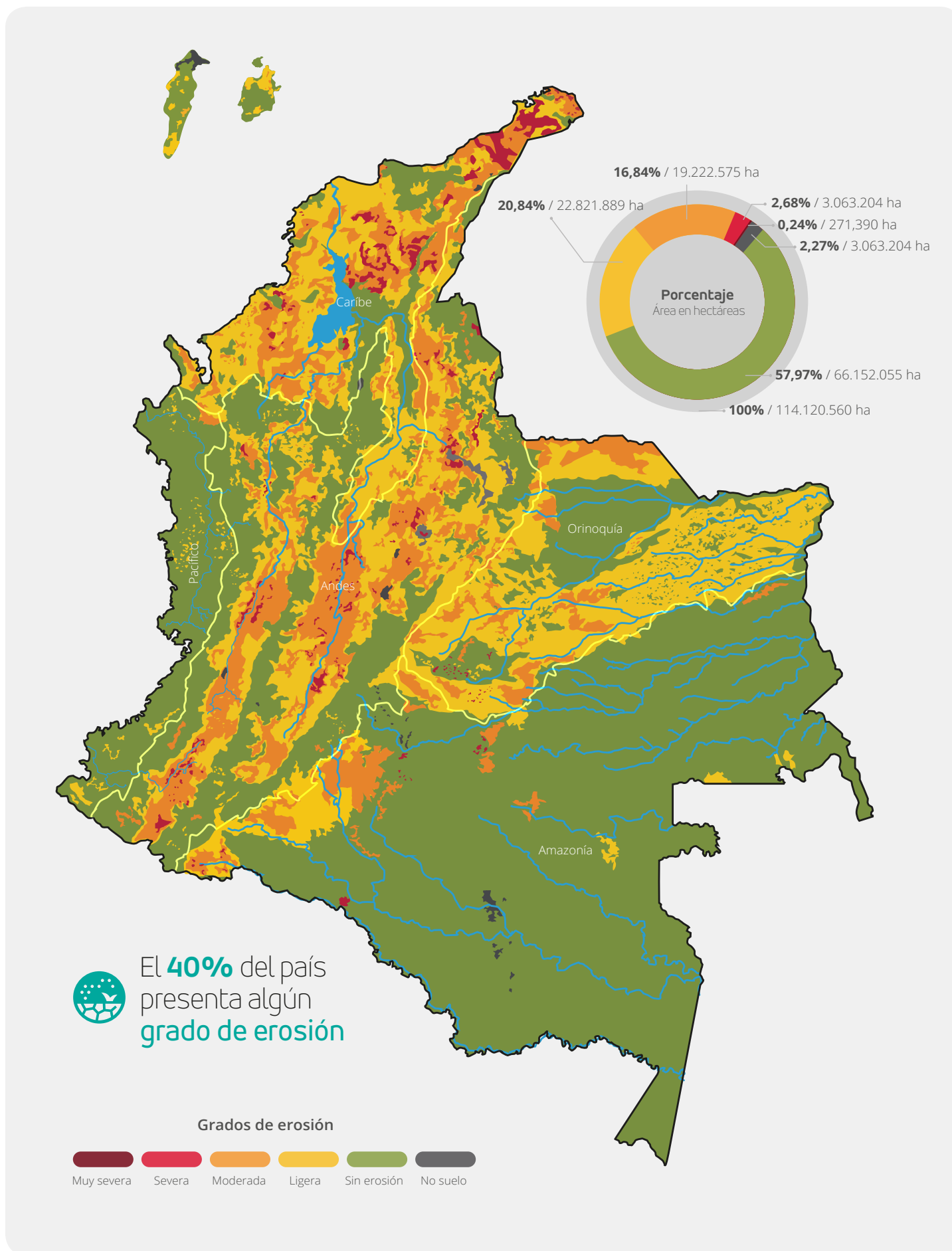
Figura 6. Zonificación de la degradación de suelos por erosión en Colombia (Ideam, 2015), (3.2.6).
