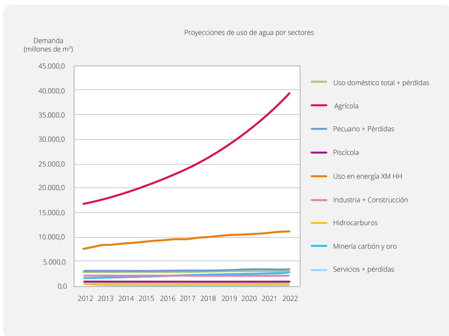
Figura 7. Proyecciones de demanda de agua por sectores 2012 -2022. (Ideam, 2015).
